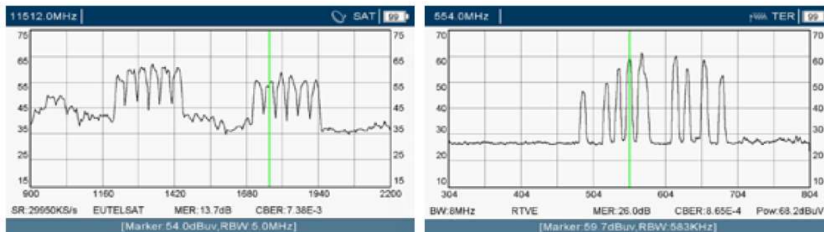
Spektrum družicového a pozemního signálu
